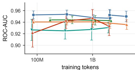
Tox21 (ROC-AUC ↑)
