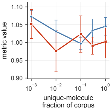
Tox21 (ROC-AUC ↑)
