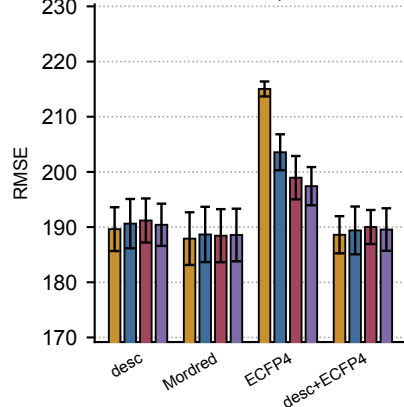
QM7 ↓
