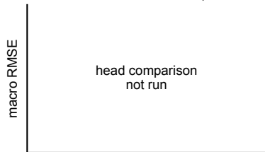
MoleculeACE ↓
