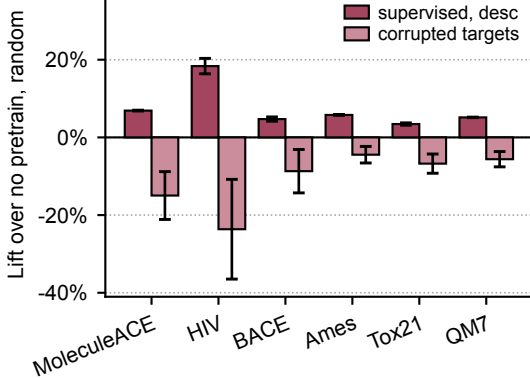
c MoIACE ↓
