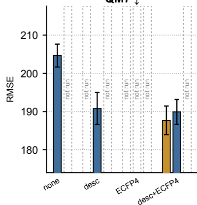
QM7 ↓
