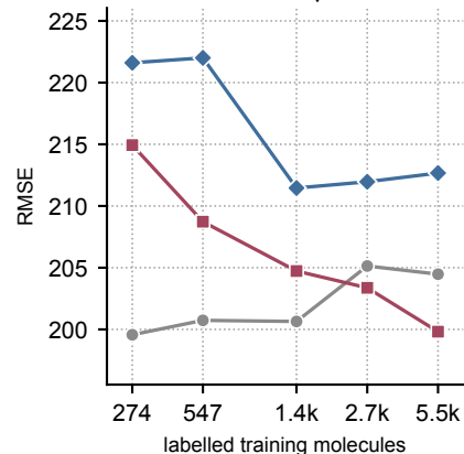
QM7 ↓
