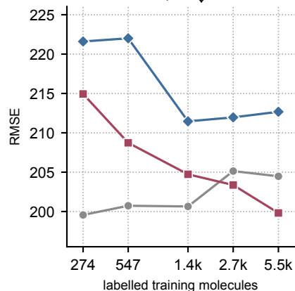
QM7 ↓
