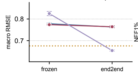
MoleculeACE ↓
