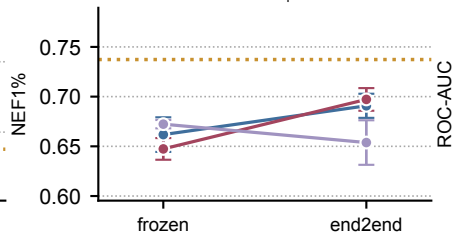
HIV ↑
