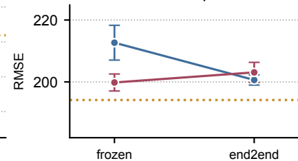
QM7 ↓
