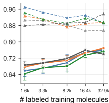
HIV (ROC-AUC ↑)
