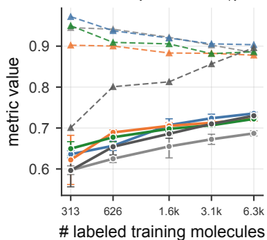
Tox21 (ROC-AUC ↑)
