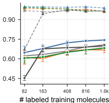
BBBP (ROC-AUC ↑)
