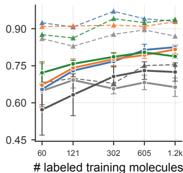
BACE (ROC-AUC ↑)
