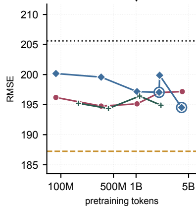
QM7 ↓
