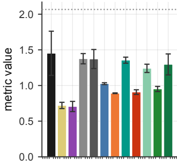
ESOL (1,128 mols) (RMSE ↓ · all scored, OOF)
