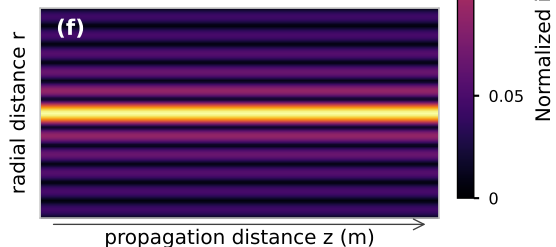
Bessel beam (ideal)
