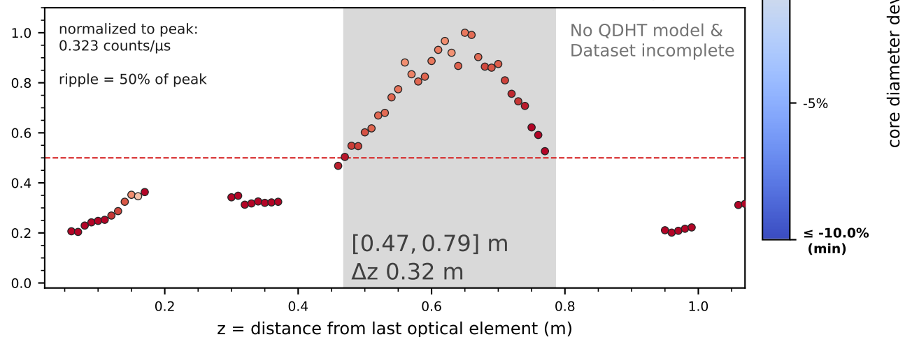
(d) Candidate #4 (Aug 6) mean core diam. = 268.1\ \mu\text{m} (+7.8% vs. ideal), FWHM = 125.6\ \mu\text{m}
