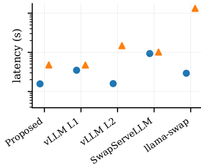
qwen-3b
