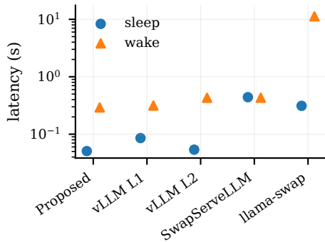
qwen-0.5b
