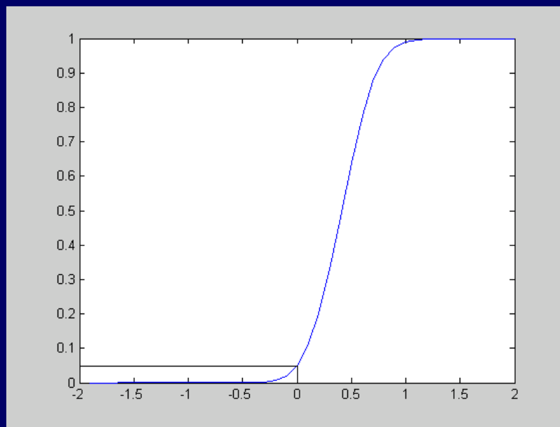
7.2.1 (a) g(\mu) 的图形
