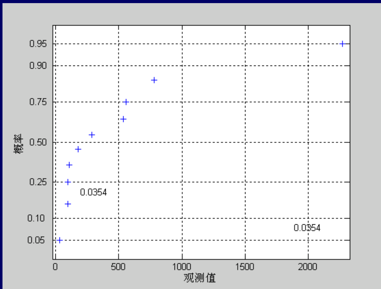
图 7.4.3 例 7.4.5 的正态概率 纸
