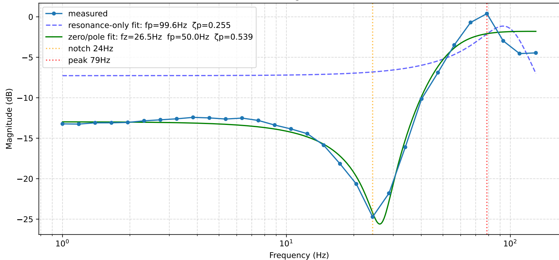
Bode Magnitude Fit
