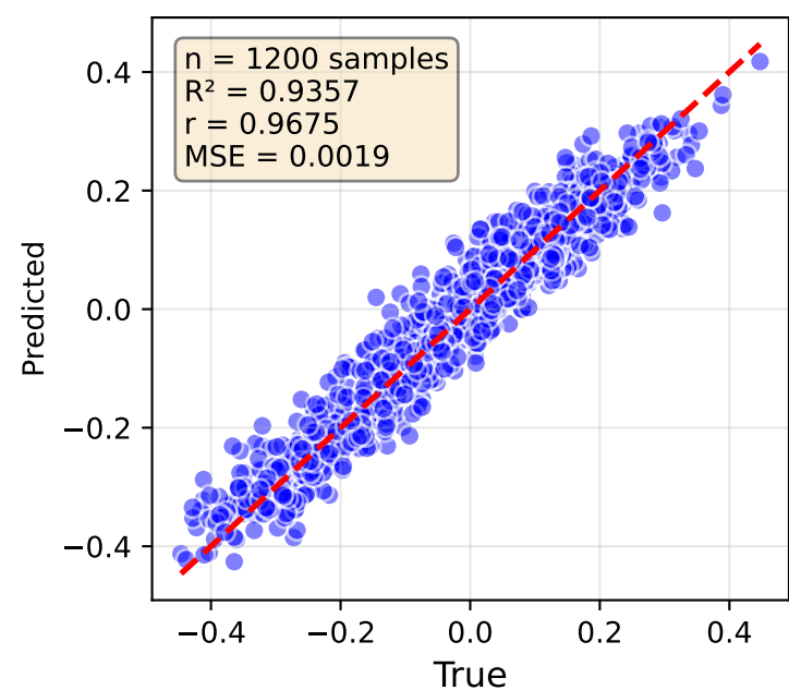
GAT - Source_Sink_Score
