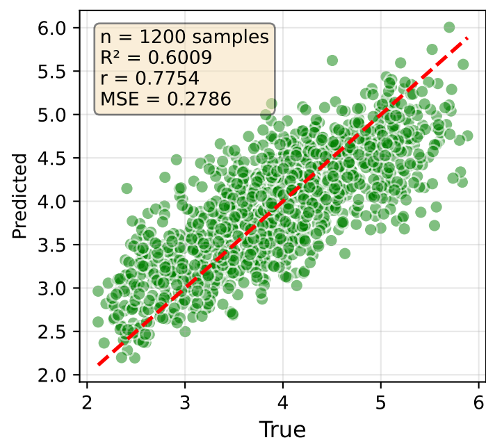
MLP - R0
