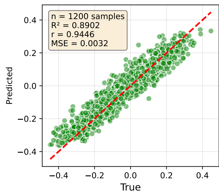
MLP - Source_Sink_Score
