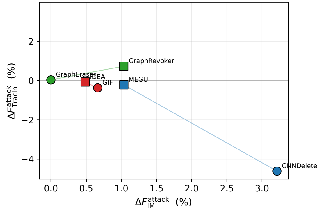
Cora · GCN
