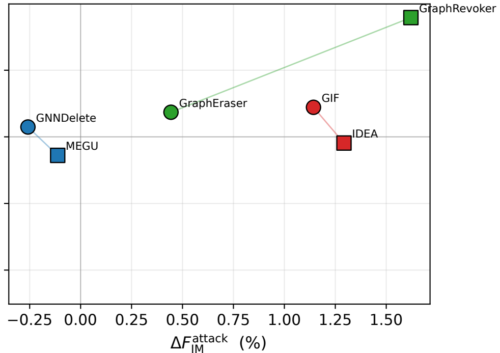
Cora · GAT
