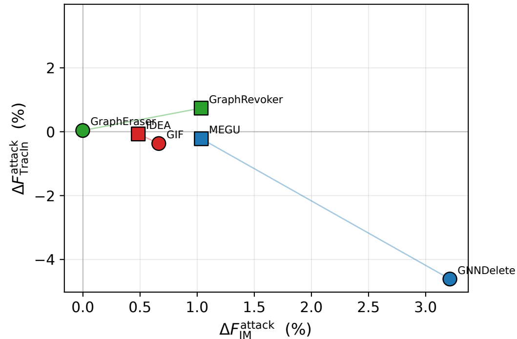
Cora · GCN
