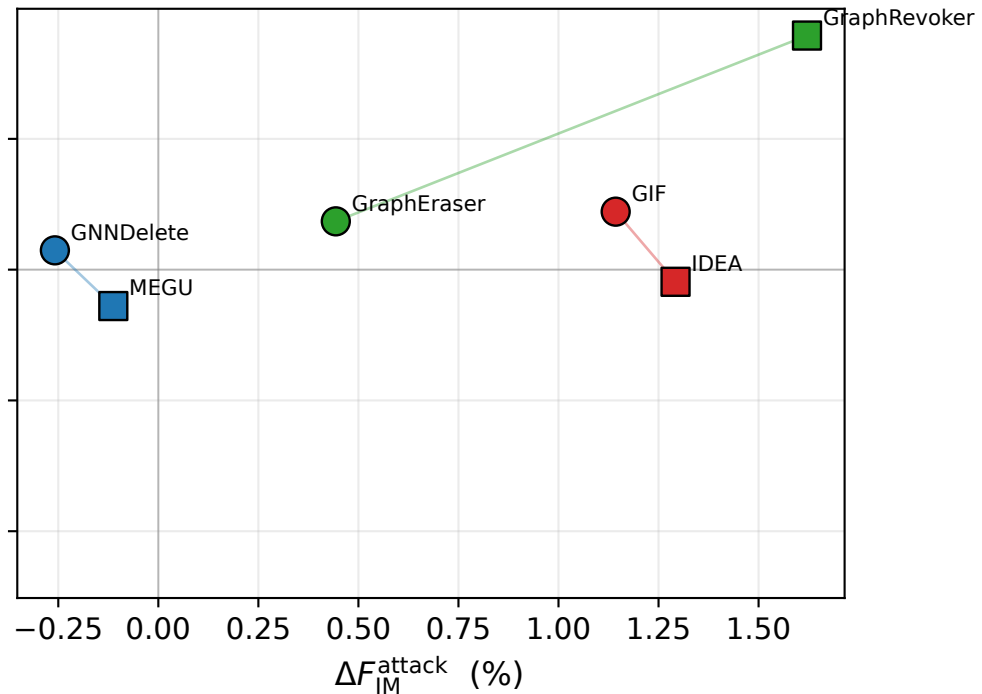
Cora · GAT
