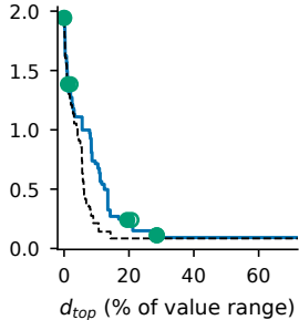
ERA5 2013/14
