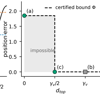
(d) trade-off
