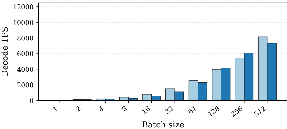
(c) Llama3 405B
