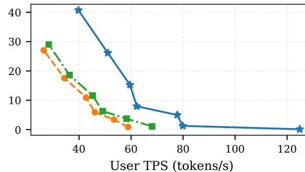
Qwen3-235B-A22B Decode
