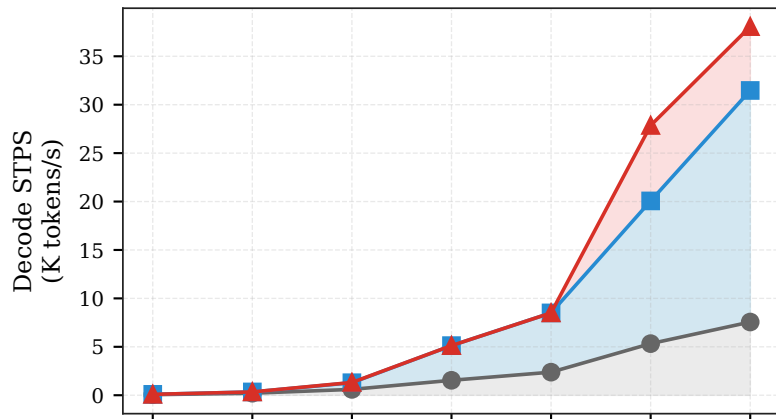
DeepSeek-V3
