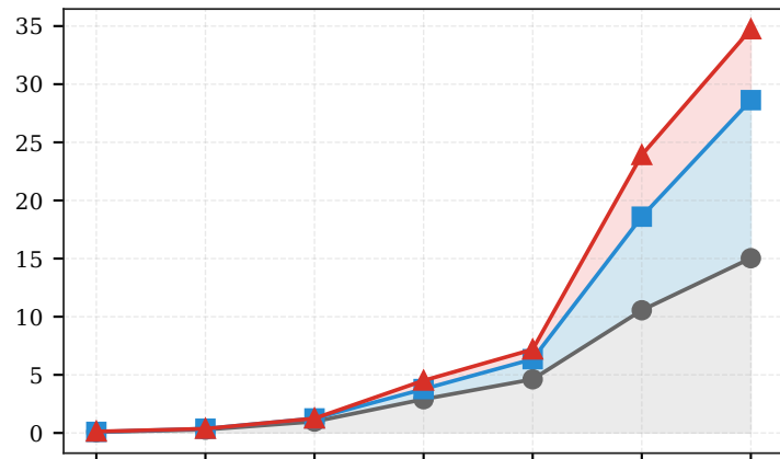
Qwen3-235B-A22B
