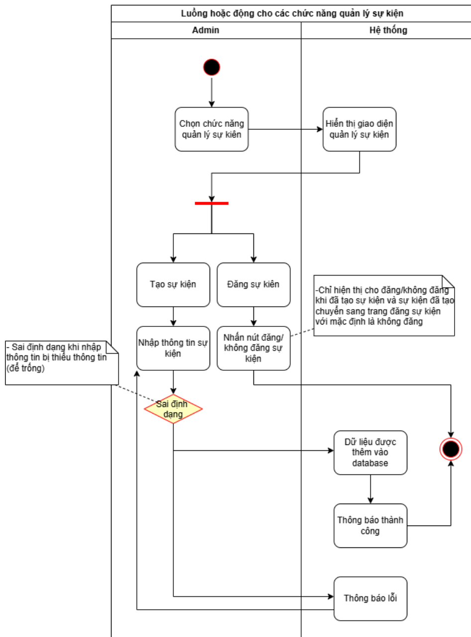
Figure 9: Hình luồng hoạt động cho chức năng quản lý sự kiện.
