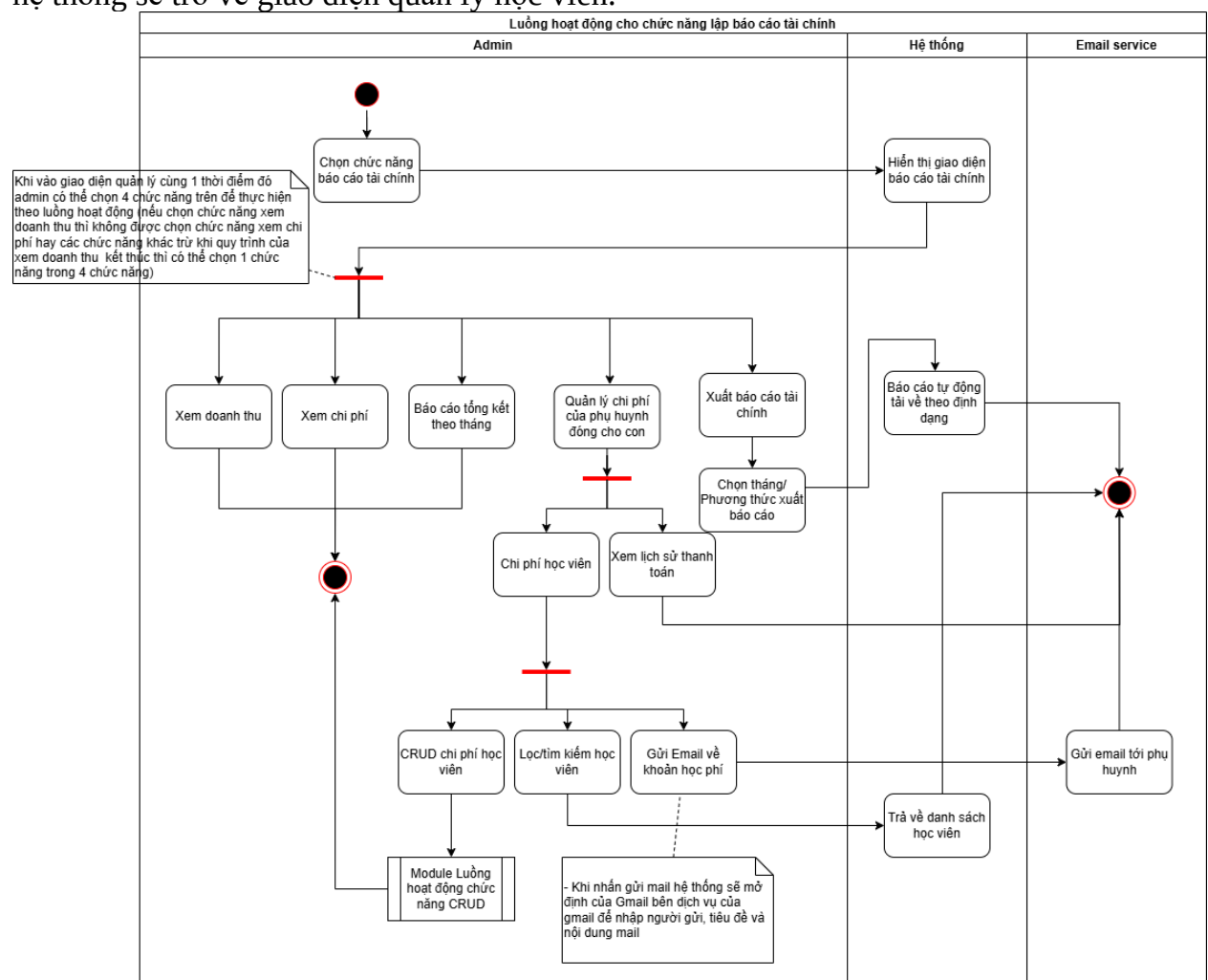
Figure 7: Hình luồng hoạt động cho chức năng lập báo cáo tài chính.
