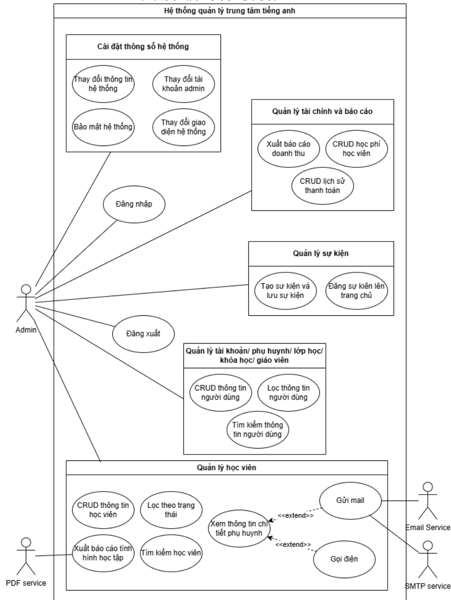
Figure 2: Hình lược đồ Use-Case.
