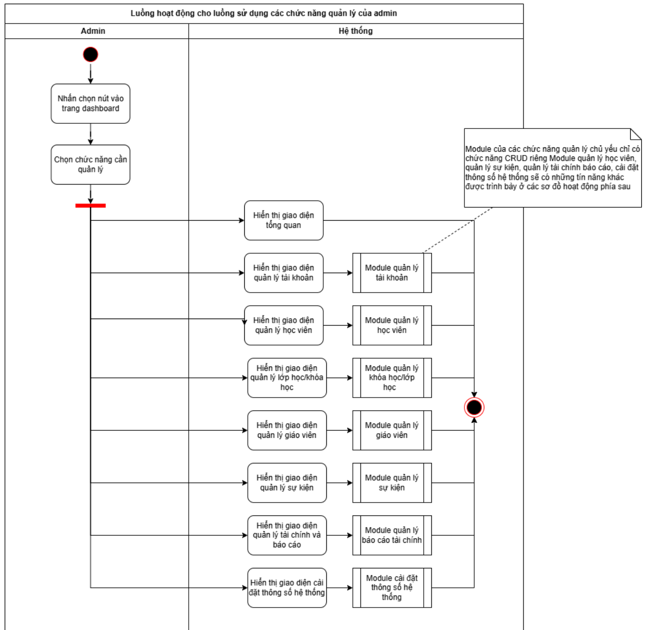
Figure 4: Hình luồng hoạt động sử dụng các chức năng chính của admin.
