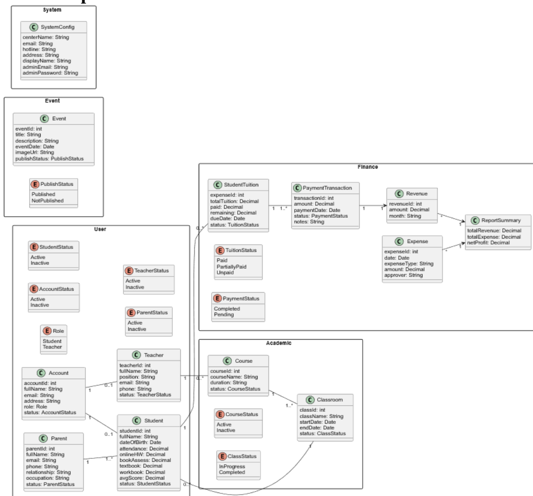
Figure 10: Hình sơ đồ lớp cho hệ thống trung tâm tiếng anh.
