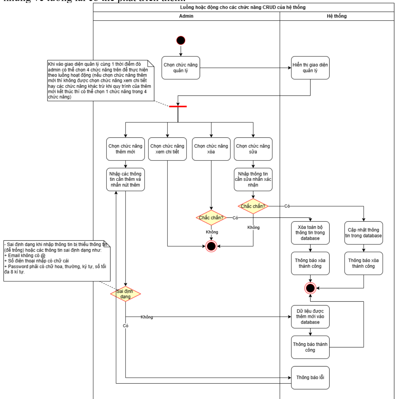
Figure 5: Hình luồng hoạt động cho các chức năng CRUD của hệ thống.
