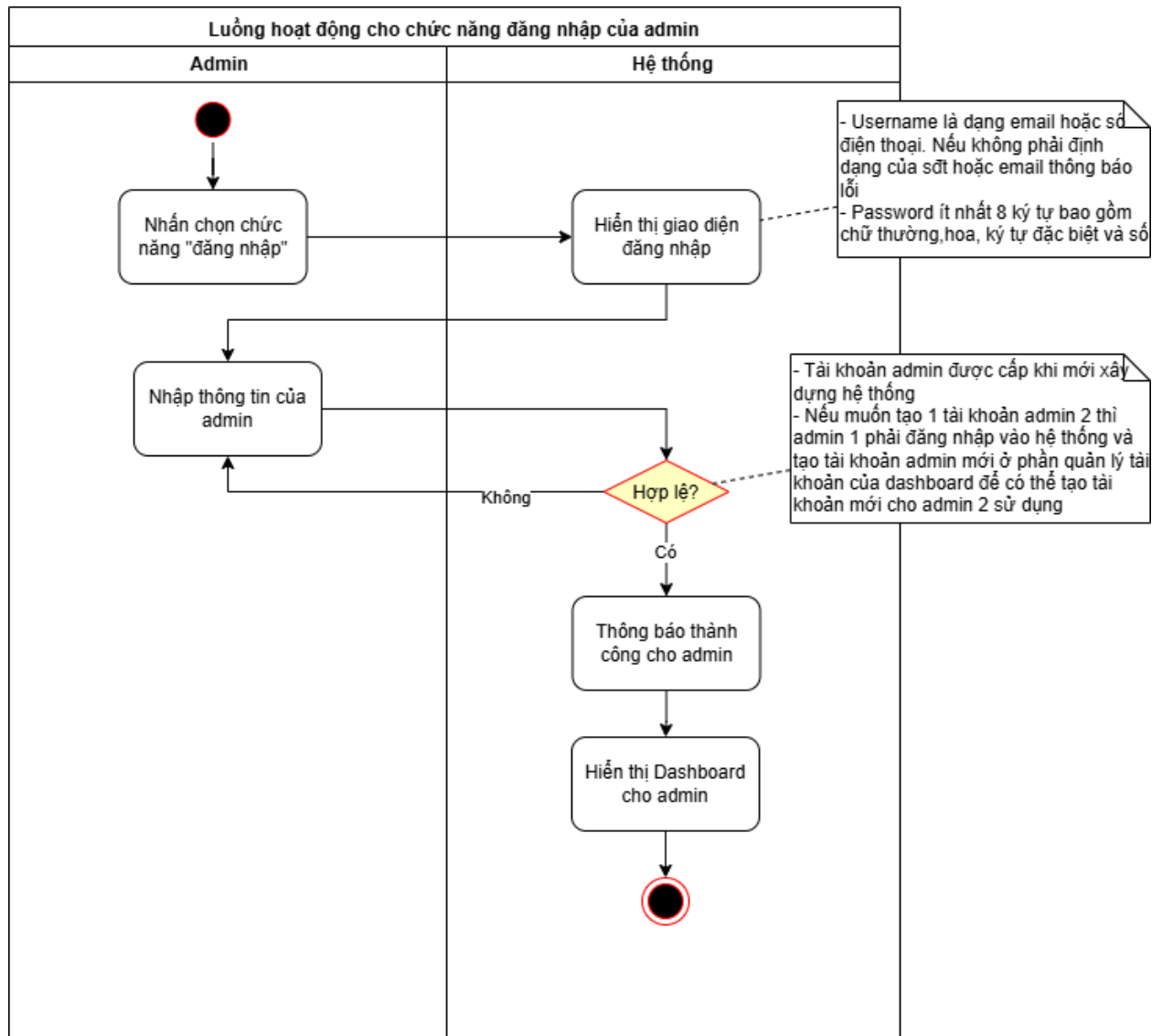
Figure 3: Hình luồng hoạt động cho chức năng đăng nhập của admin
