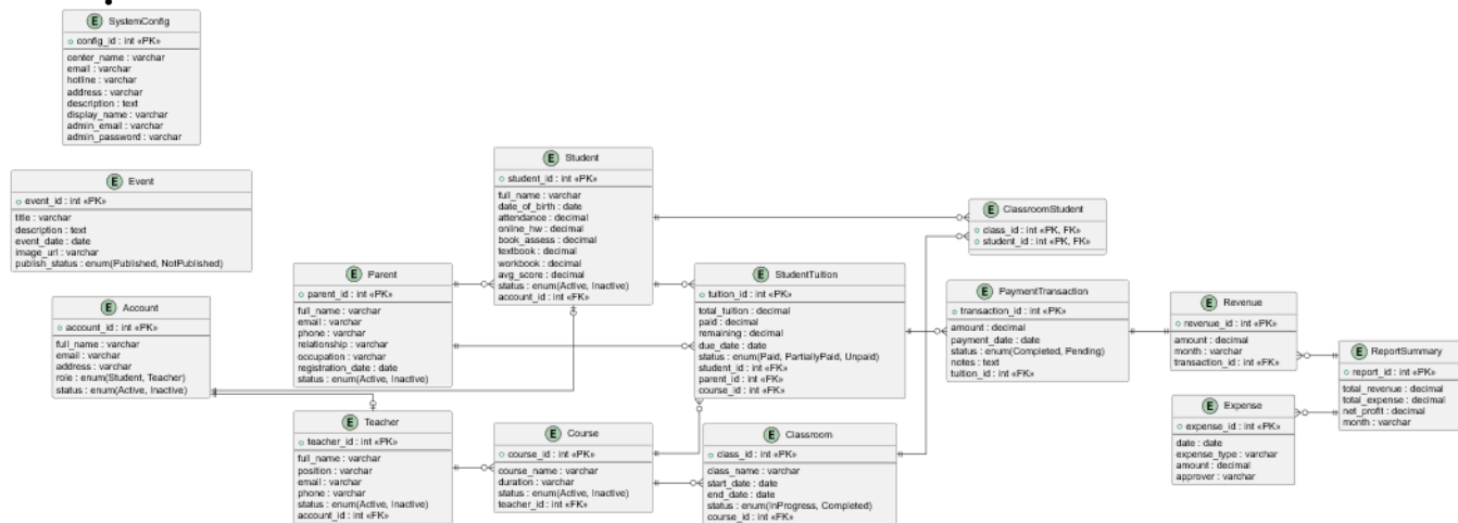
Figure 11: Hình lược đồ CSDL cho hệ thống trung tâm tiếng anh.
