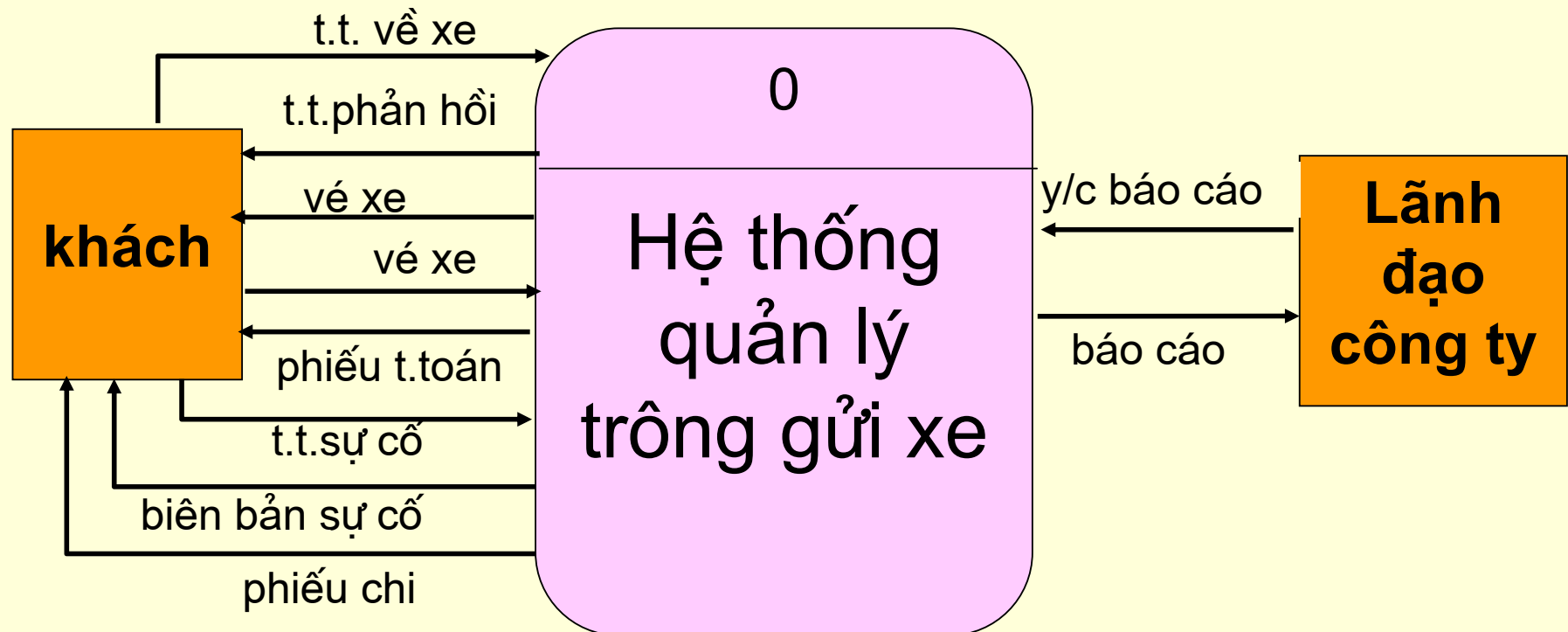
Hình 1. Biểu đồ ngữ cảnh của hệ thống
