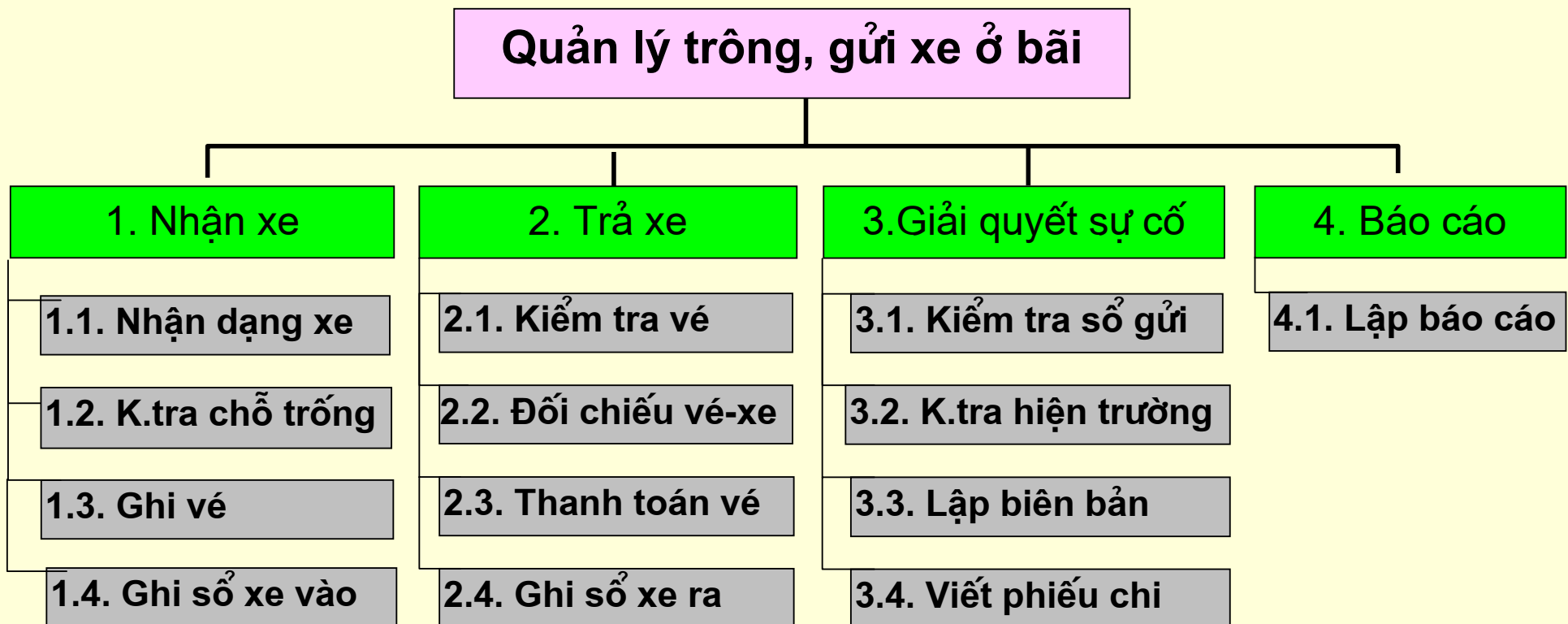
Hình 2. Biểu đồ phân rã chức năng hoạt động trông gửi xe ở bãi
