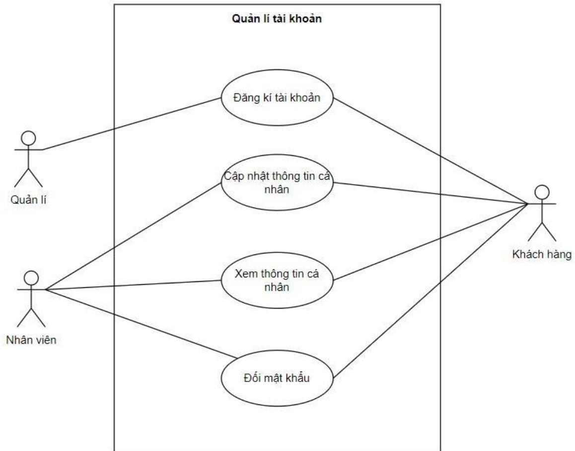
Hình 3: Phân rã use case chức năng quản lý tài khoản
