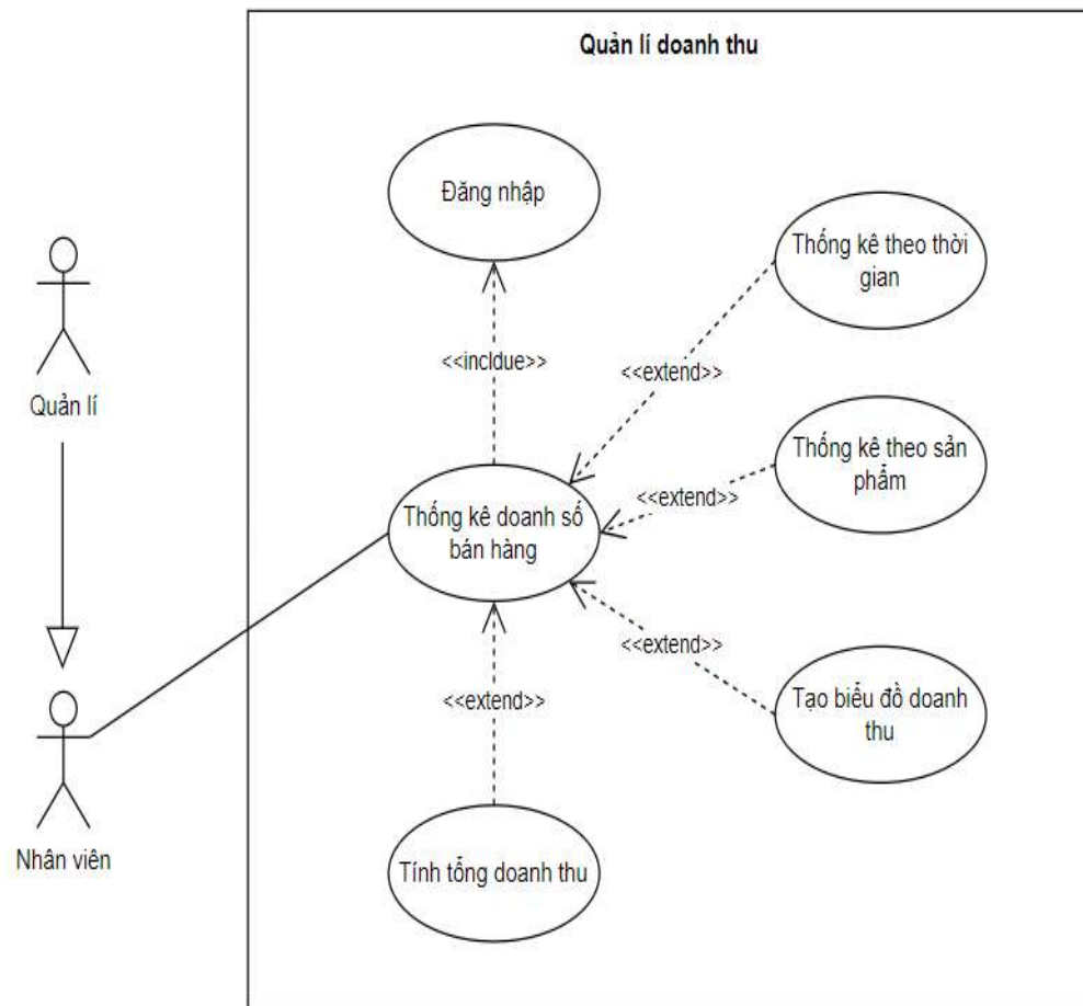
Hình 6. Phân rã chức năng quản lý doanh thu
