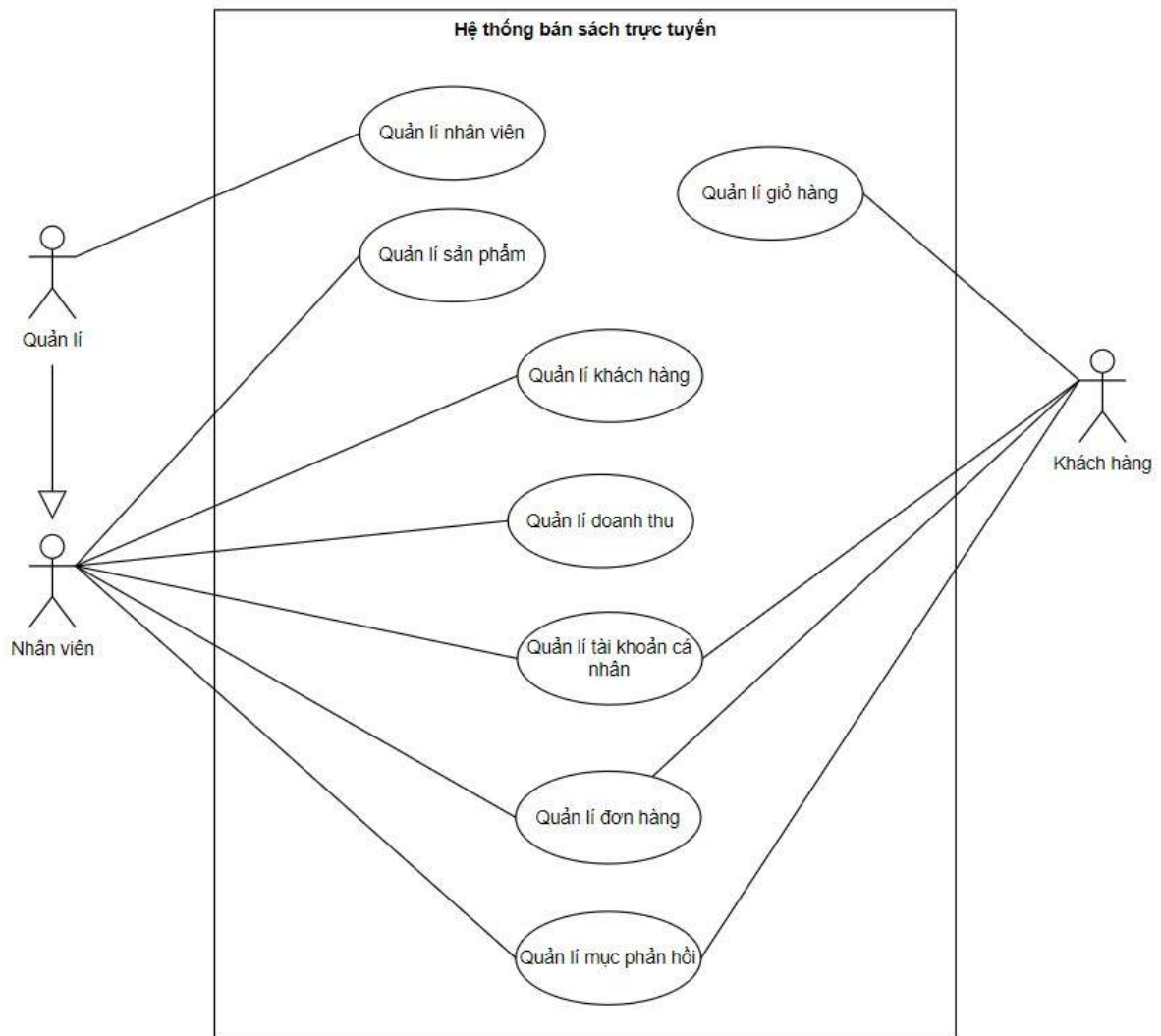
Hình 1. Biểu đồ use case tổng quát
