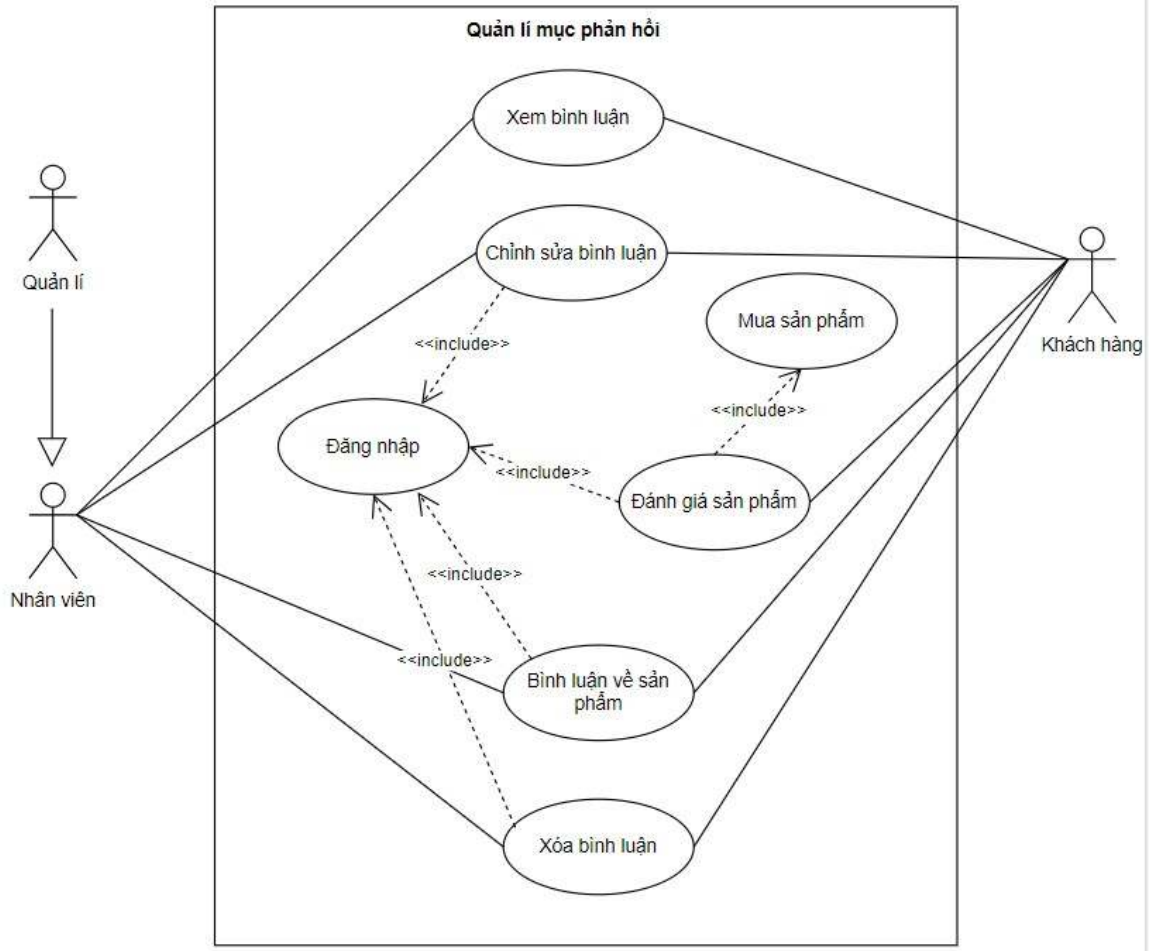
Hình 9. Phân rã chức năng quản lý mục phản hồi
