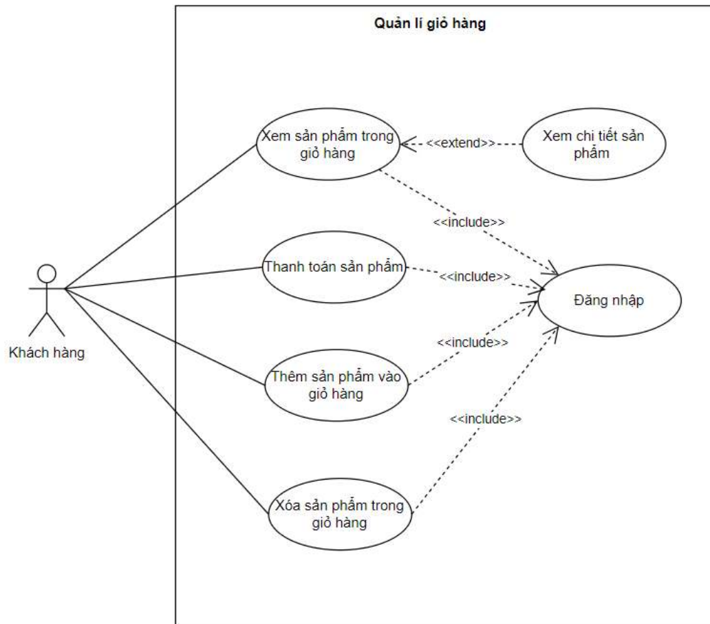
Hình 5. Phân rã chức năng quản lý giỏ hàng
