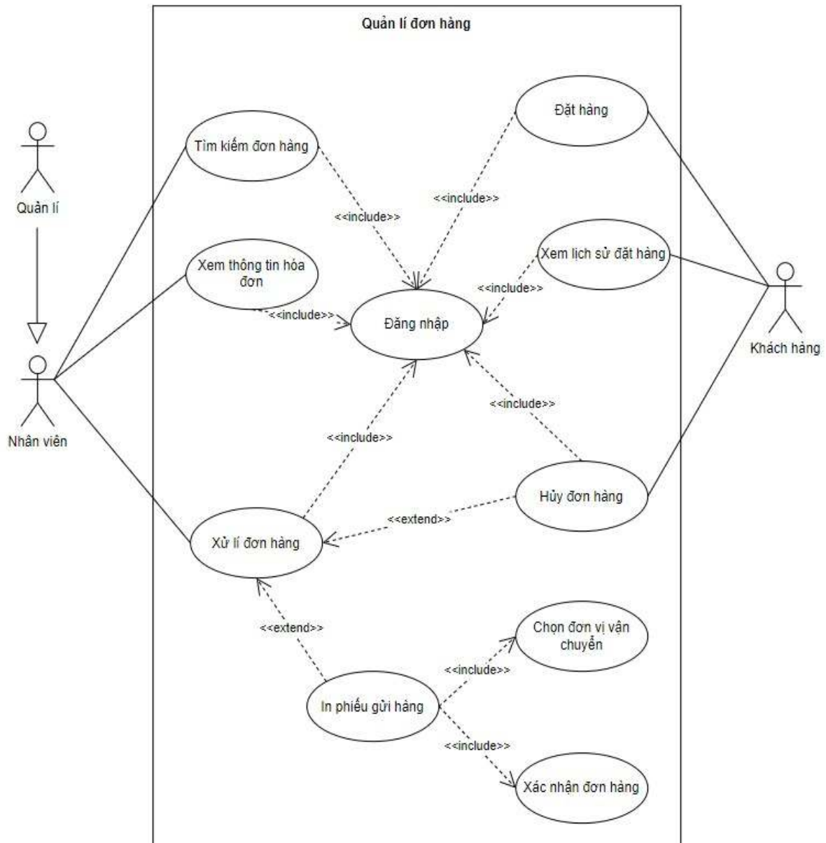
Hình 4. Phân rã chức năng quản lý đơn hàng
