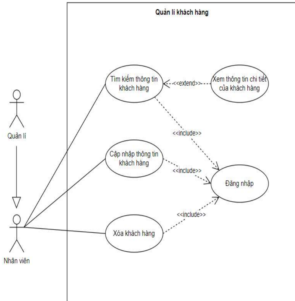
Hình 8. Phân rã chức năng quản lý khách hàng
