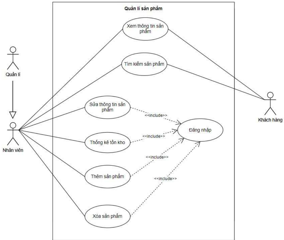
Hình 2: Phân rã use case quản lí sản phẩm
