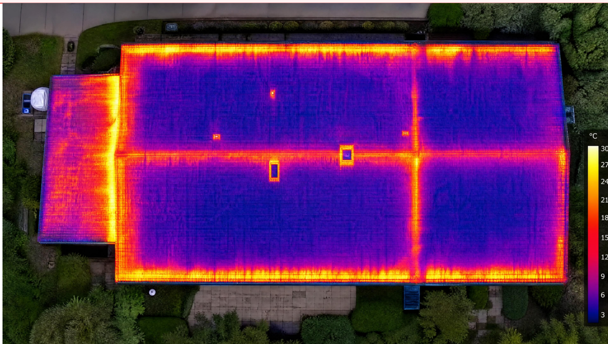
Simulation visuelle des zones de déperdition – à confirmer par diagnostic sur site
