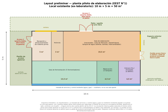
Layout preliminar del local existente (10 m × 5 m = 50 m²) para la planta piloto de EEST N°1
