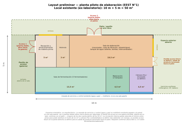
Layout preliminar del local existente ( 10\text{ m} \times 5\text{ m} = 50\text{ m}^2 ) para la planta piloto de EEST N°1
