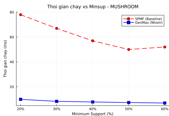
Hình 3: Thời gian chạy trên Mushroom
