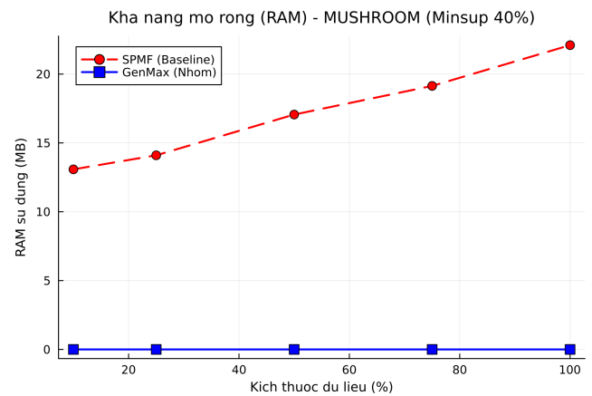
Hình 15: Khả năng mở rộng (Bộ nhớ)
