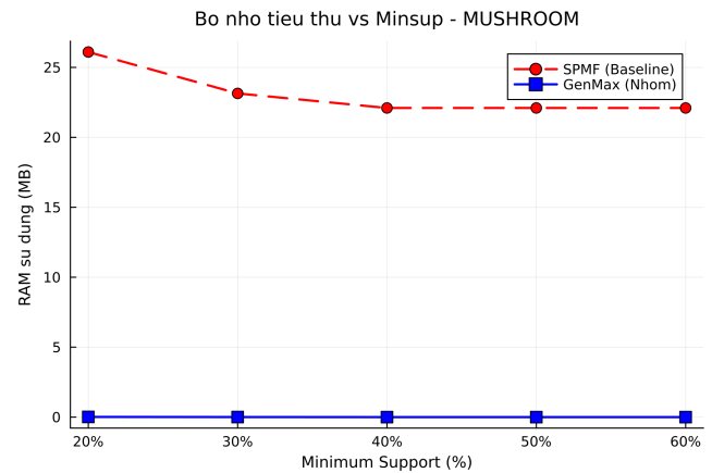
Hình 11: Bộ nhớ trên Mushroom
