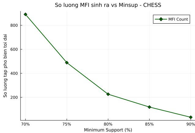
Hình 6: Số MFI sinh ra trên Chess
