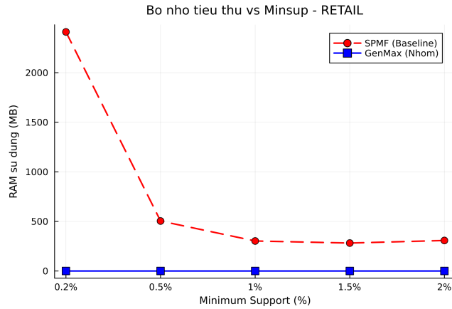
Hình 12: Bộ nhớ trên Retail
