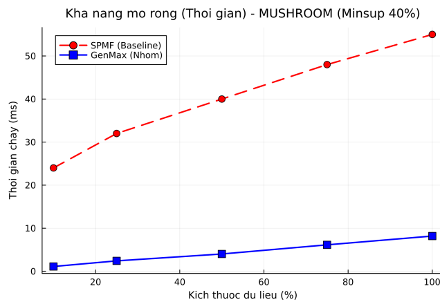
Hình 14: Khả năng mở rộng (Thời gian)
