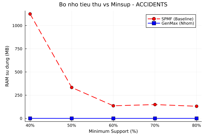
Hình 13: Bộ nhớ trên Accidents
