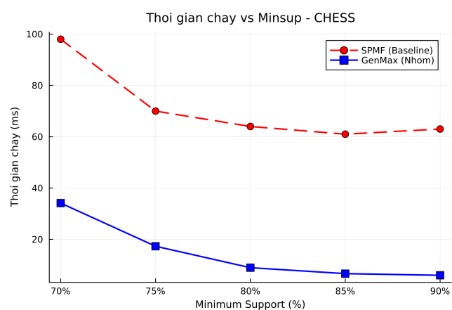
Hình 2: Thời gian chạy trên Chess
