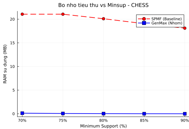
Hình 10: Bộ nhớ trên Chess
