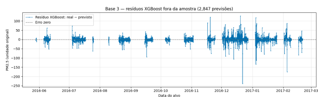
Base 3: Resíduos XGBoost fora da amostra. Fonte: notebooks/base_03-grupo3_XGBoost.ipynb#cell-14.
