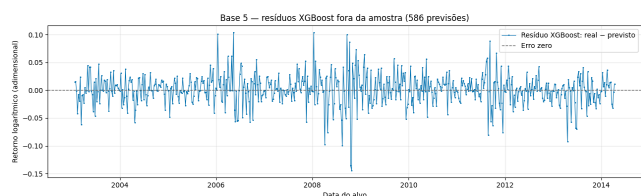
Base 5: Resíduos XGBoost fora da amostra. Fonte: notebooks/base_05-grupo5_XGBoost.ipynb#cell-14.
