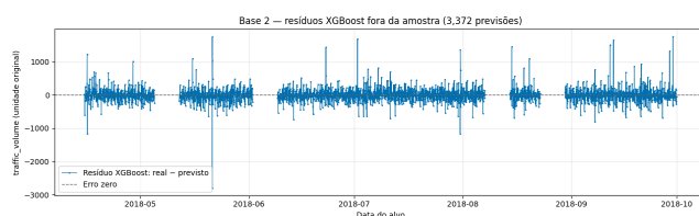
Base 2: Resíduos XGBoost fora da amostra. Fonte: notebooks/base_02-grupo2_XGBoost.ipynb#cell-14.
