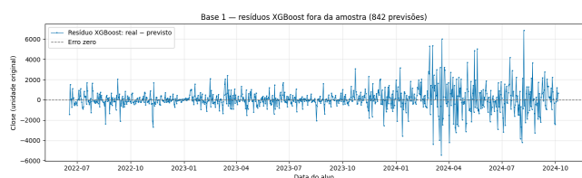
Base 1: Resíduos XGBoost fora da amostra. Fonte: notebooks/base_01-grupo1_XGBoost.ipynb#cell-14.
