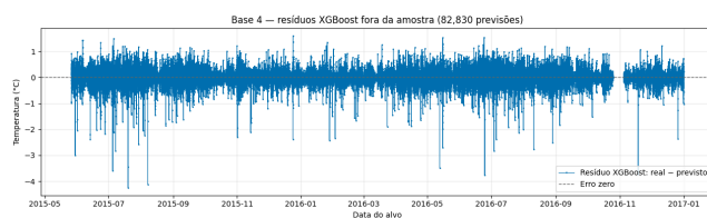
Base 4: Resíduos XGBoost fora da amostra. Fonte: notebooks/base_04-grupo4_XGBoost.ipynb#cell-14.
