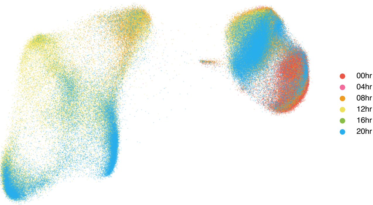
acaA - pkaC
