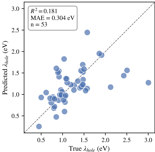
SchNet FedAvg (E14): Client D LOOCV
