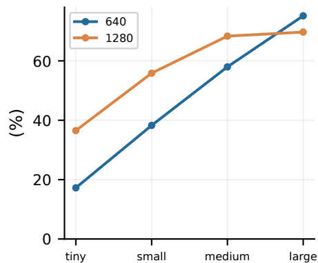
YOLOv8s | CLEAN: size AR
