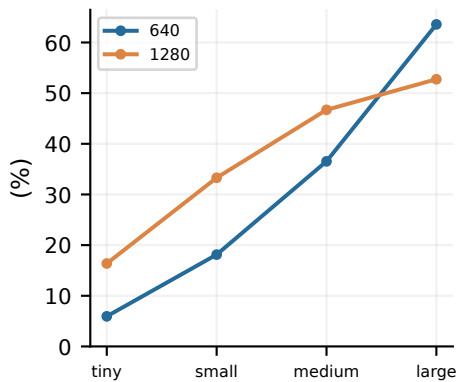
YOLO26s | CLEAN: size AP
