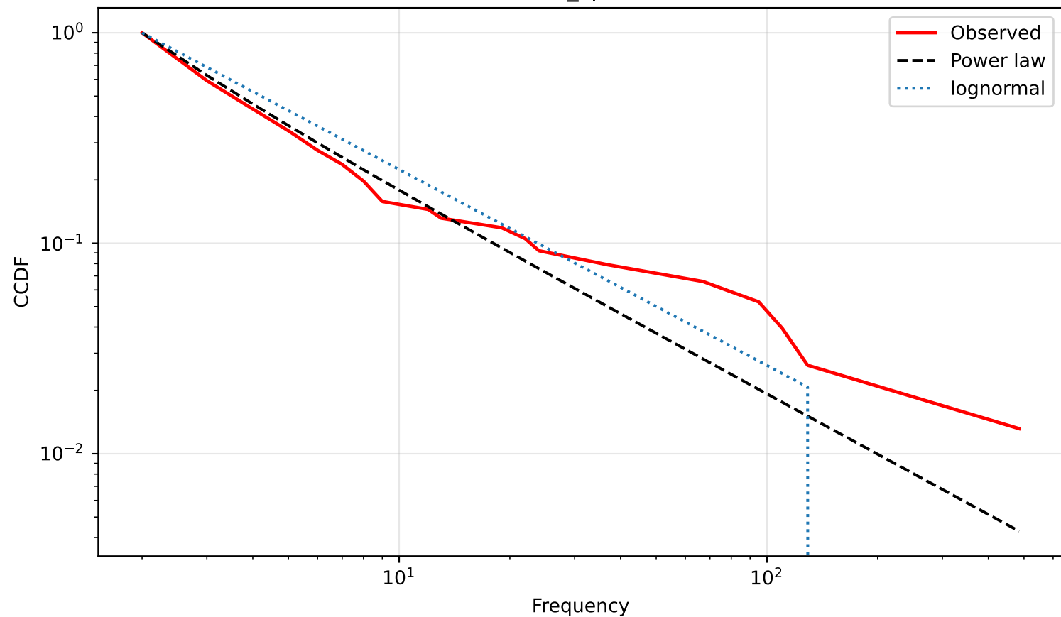
BPIC13_cp CCDF
