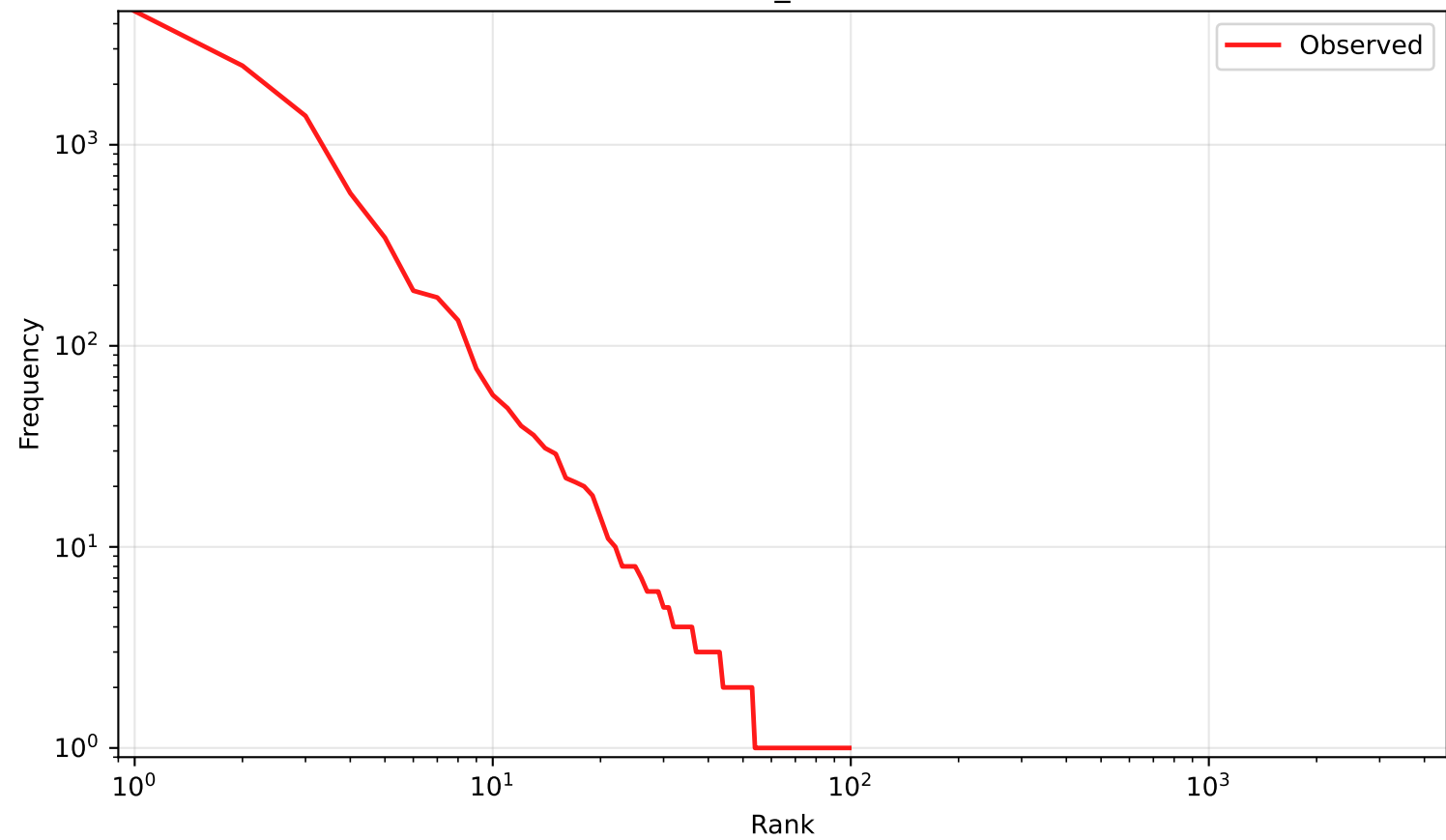
BPIC20_dd RFC
