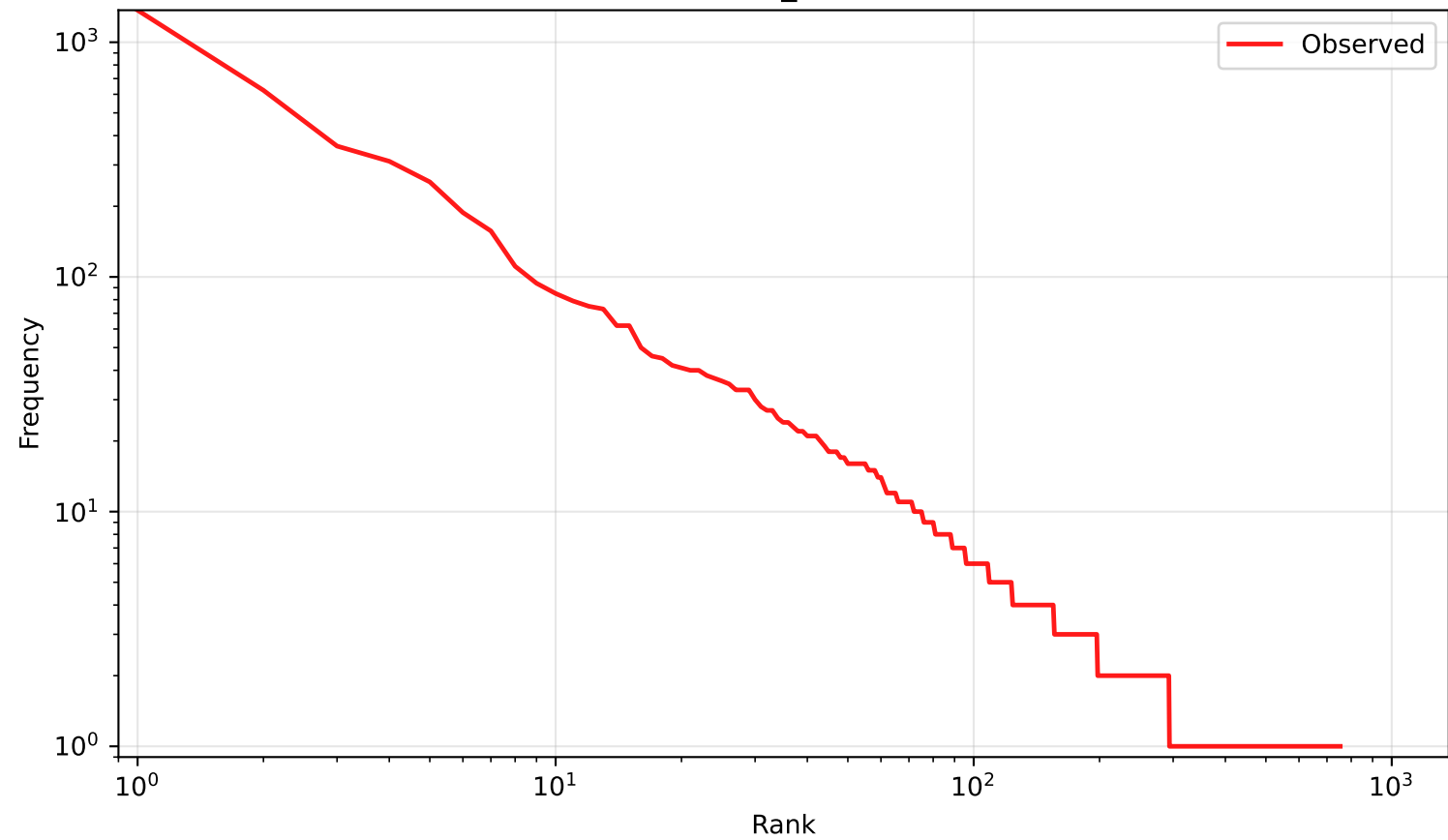
BPIC20_id RFC
