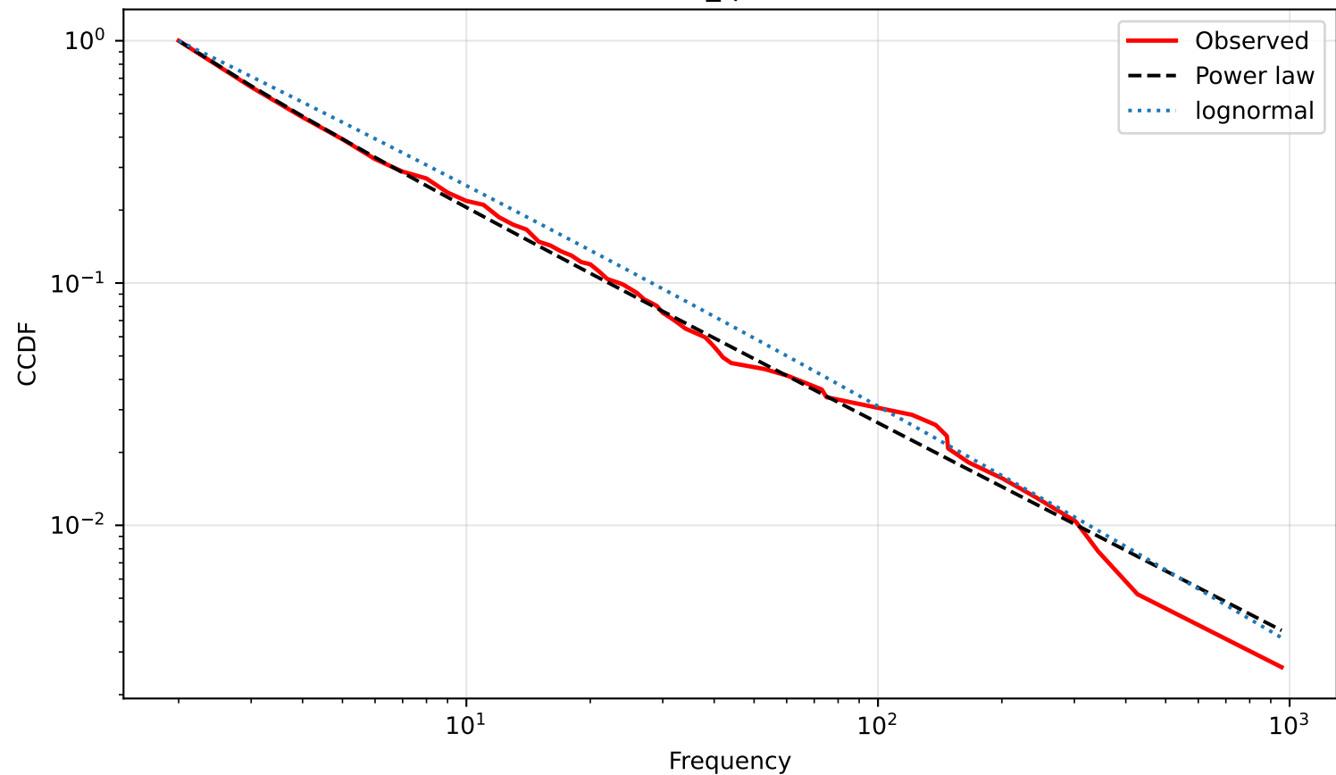
BPIC20_tpd CCDF
