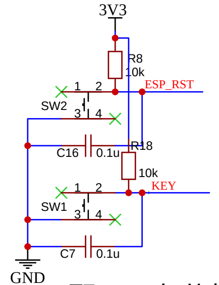
配网、复位按键
