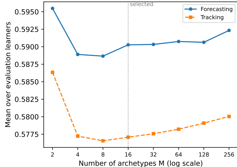
Held-out NLL
