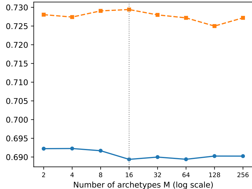
Held-out AUC
