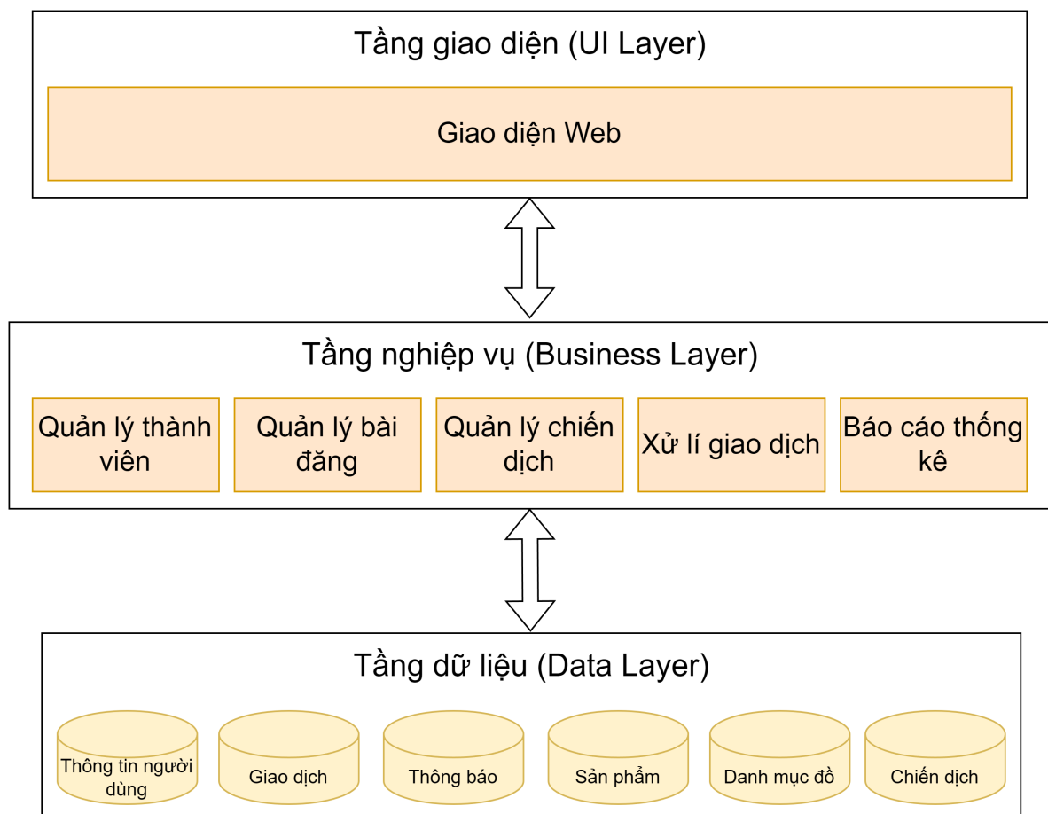
Hình 2.1.1: Kiến trúc tổng quan
