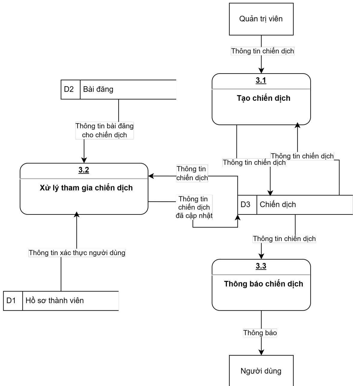
Hình 2.5.3: Quản lý chiến dịch
