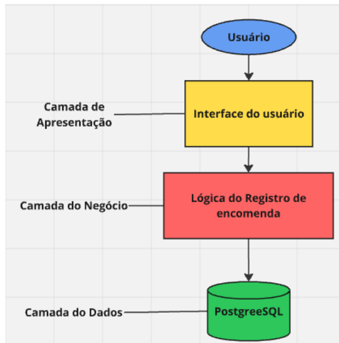
Diagrama 1 - Arquitetura de sistema
