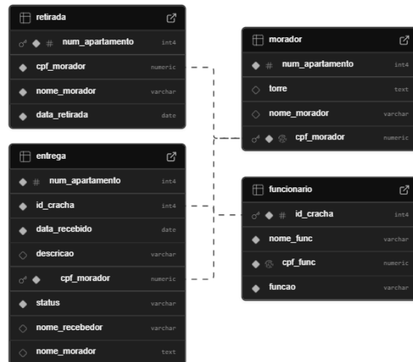
Diagrama 3 - Estrutura das tabelas
