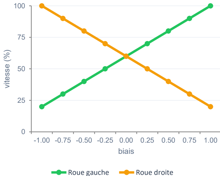
Vitesse des roues selon le biais
