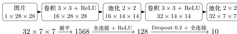
图 2: 自己绘制的 CNN 结构图。卷积核提取局部形状，池化缩小特征图，末端输出类别分数。
