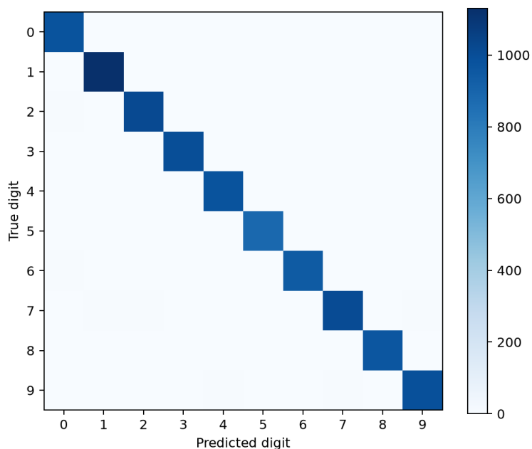
图 4: 增强 CNN 的 MNIST 测试集混淆矩阵，纵轴是真实类别，横轴是预测类别。
