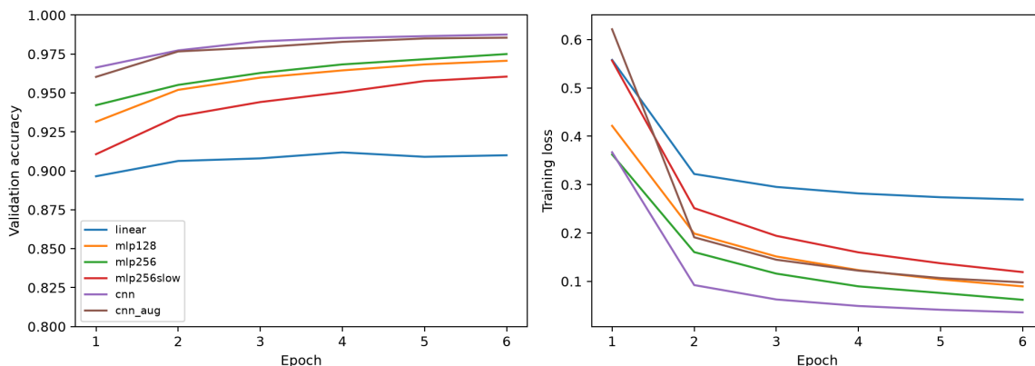
图 3: 六组实验的逐轮验证准确率和训练损失，由本实验代码绘制。
