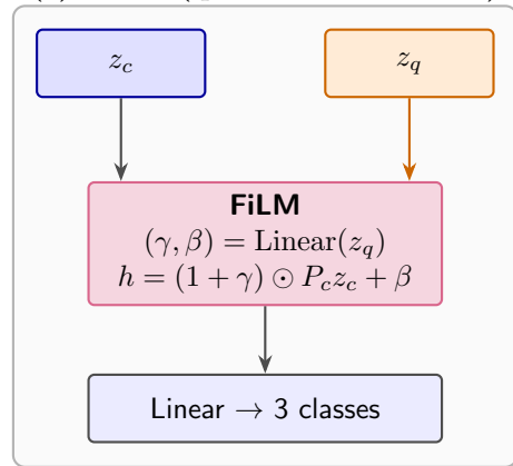
(c) FiLM (quantum modulates)
