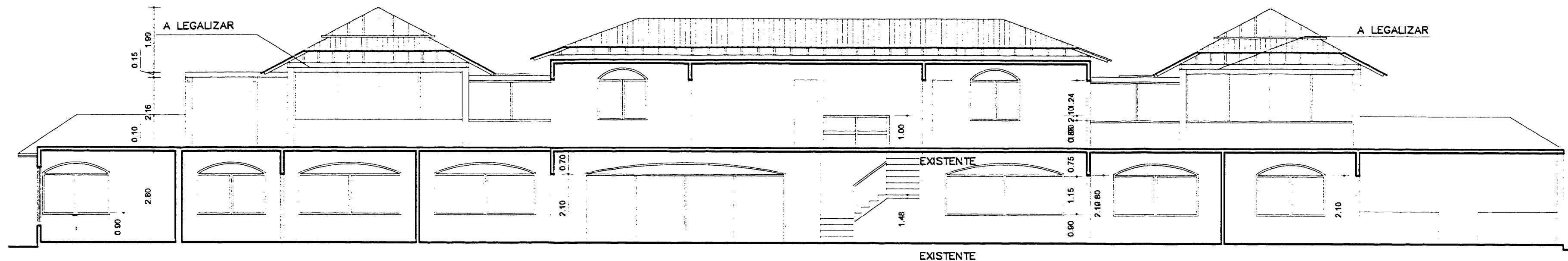
CORTE AA ESCALA = 1/100
