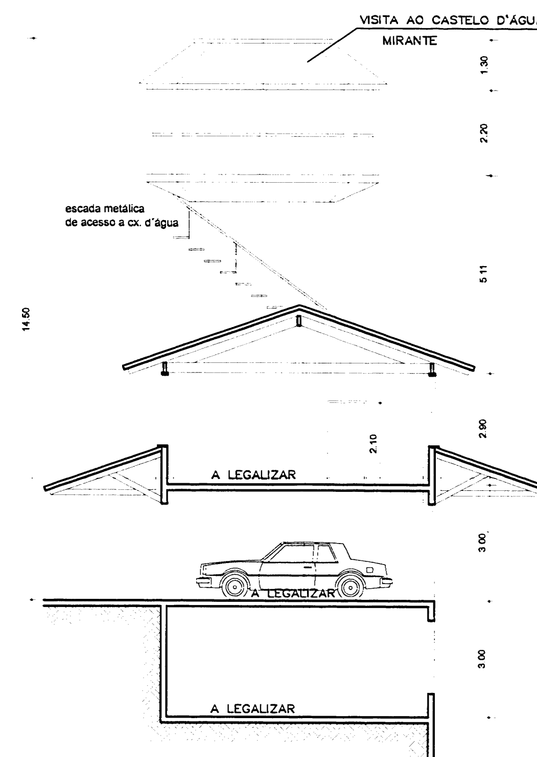
CORTE DD ESCALA = 1/100
