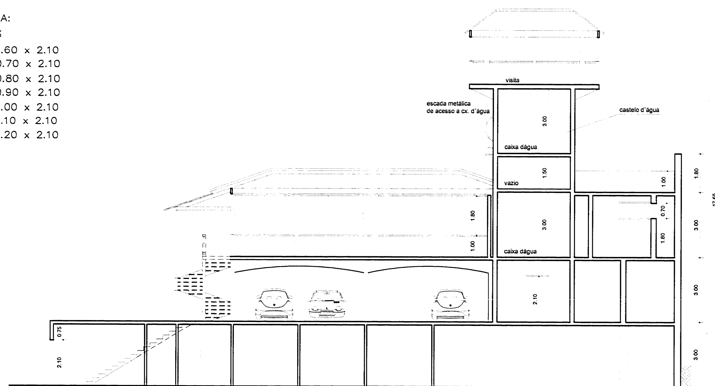
CORTE CC ESCALA = 1/100
