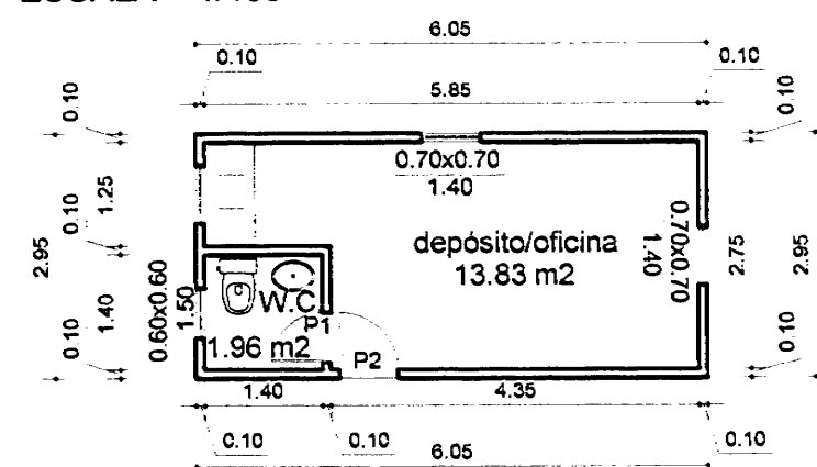
PLANTA BAIXA - DEPÓSITO ÁREA = 17.84 m² ESCALA = 1/100
