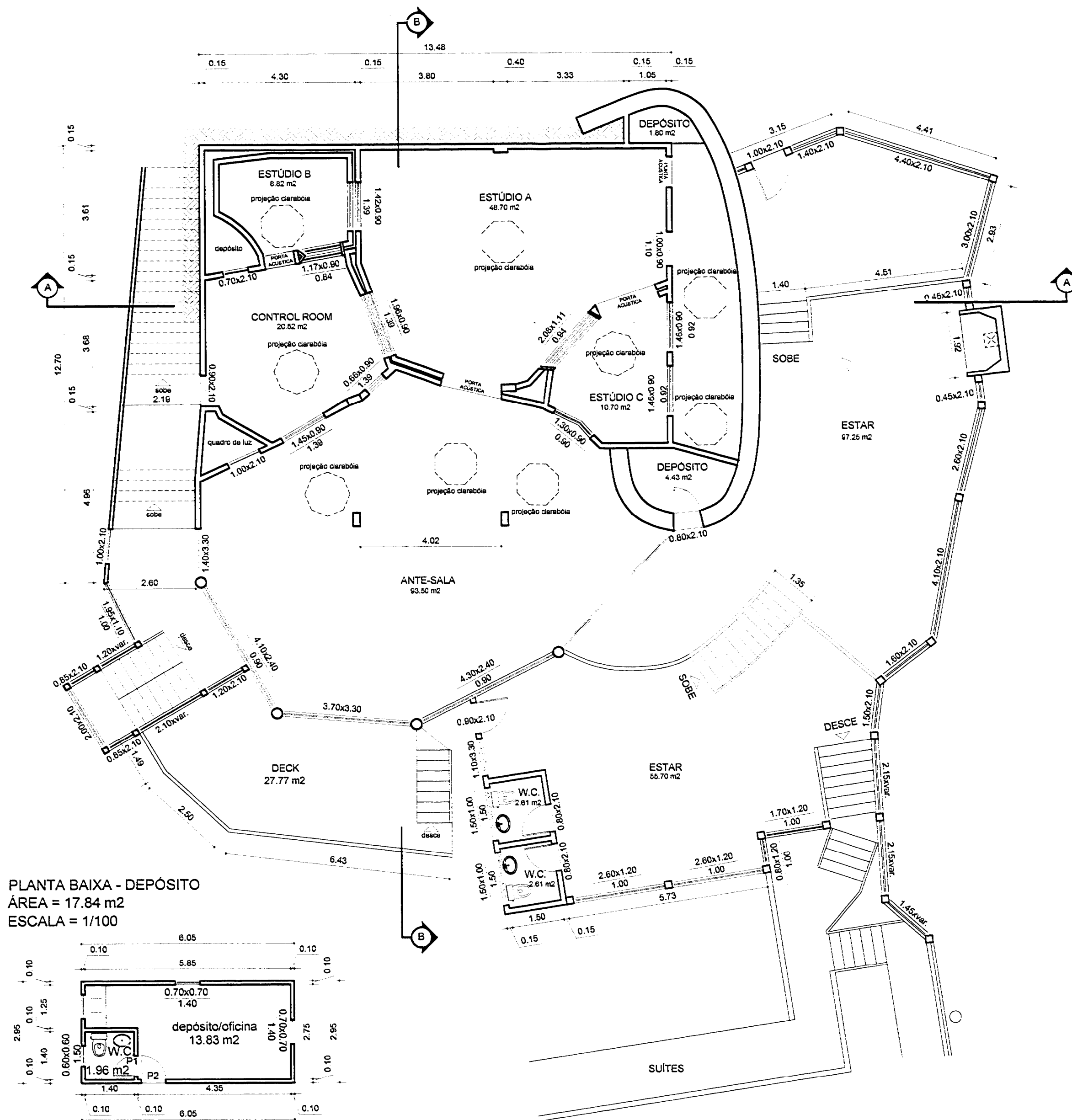
PLANTA BAIXA - ESTÚDIO / ESTAR ÁREA = 408.27 m² ESCALA = 1/100
