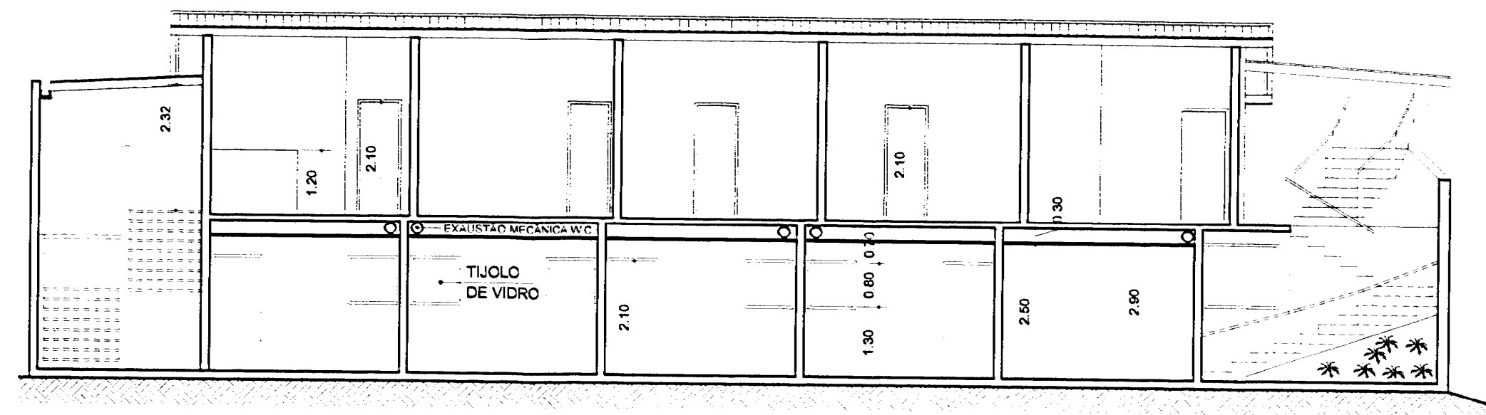
CORTE C-C ESCALA = 1/100
